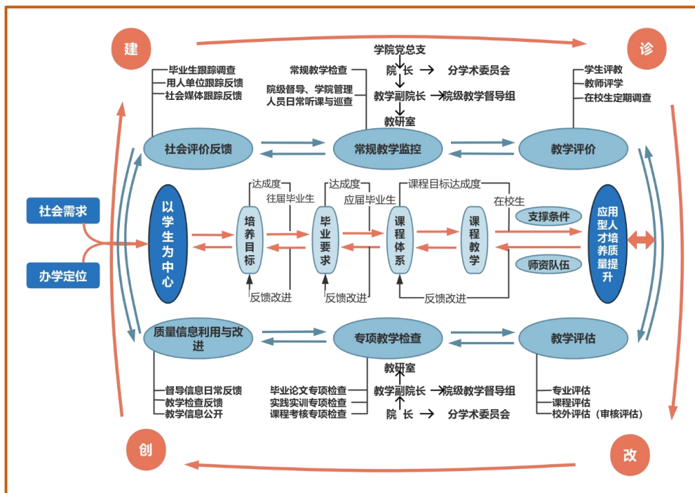
图3 “建、诊、创、改” 闭环式教学质量保障体系
